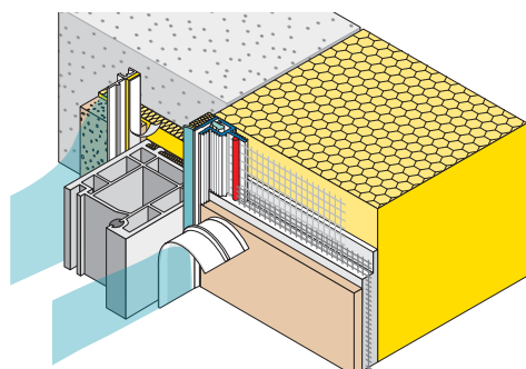
Lišta s tkaninou teleskopická s jazýčkem
