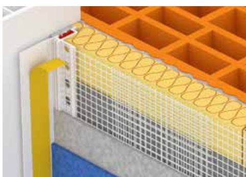
Lišta s tkaninou FAP Compact 3D PRO
