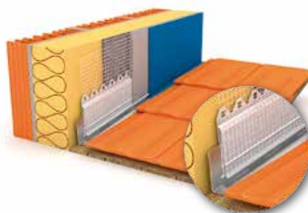
Ukončovací profil napojení oplechování k ETICS (F050-250)
