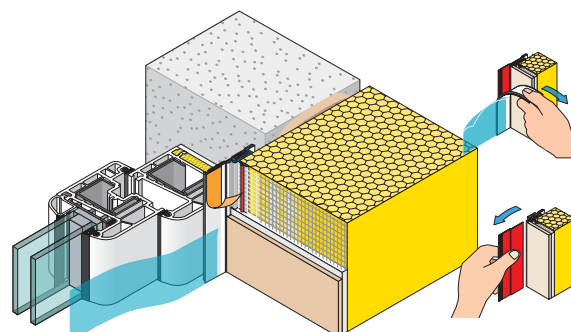
Lišta s tkaninou PUR-FIX-pro
